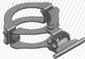
Bild 30: Zwischenverankerung, Typ: AIO-SZH-20
