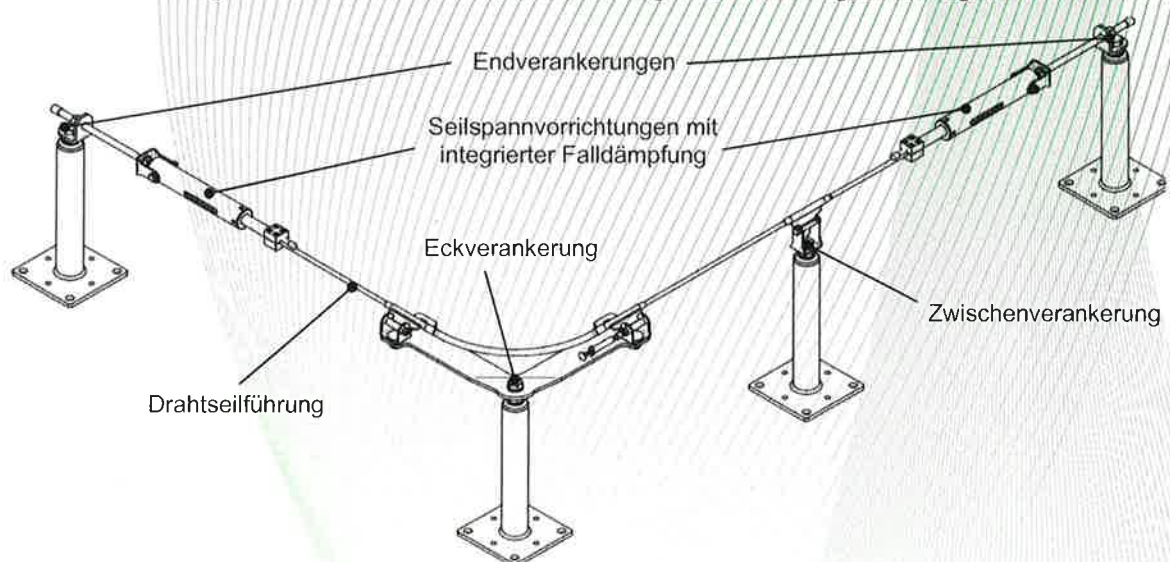
Bild 1: Anwendungsbeispiel der Anschlagereinrichtung, Typ: ALLinONE
