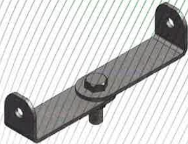
Bild 12: Endverankerung, Typ: AIO-EB-14
