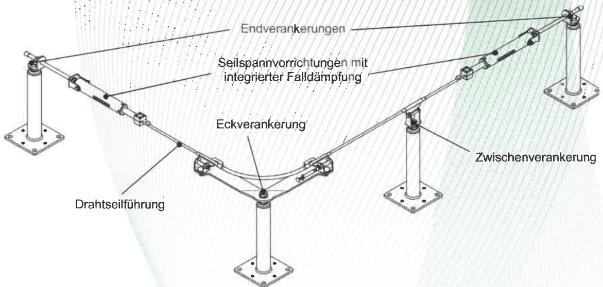
Bild 1: Anwendungsbeispiel der Anschlageinrichtung, Typ: ALLinONE
