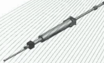
Bild 24: Seilspanner Typ: AIO-ENDS-10
