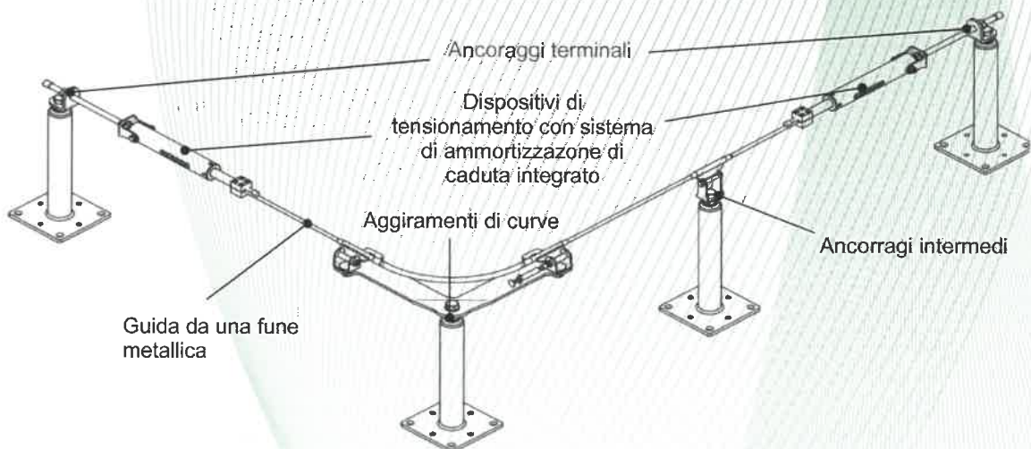
Fig. 1: Esempio di applicazione del dispositivo di ancoraggio, tipo: ALLinONE
