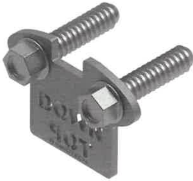
Photo 18 : Terminaison de rail Type : TAURUS-EA-12
