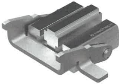
Photo 16 : Terminaison de rail Type : TAURUS-EA-11
