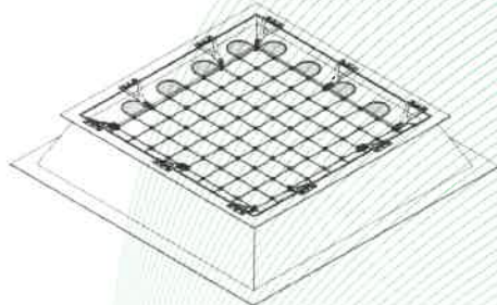
Ilustración 1: Sistema de protección contra caídas, tipo: LIGHT-FLEX - modelo cerrado
