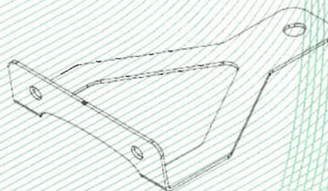
Ilustración 5: Portador canteado del sistema de protección contra caídas, tipo: LIGHT-FLEX / LIGHT-FLEX-RWA
